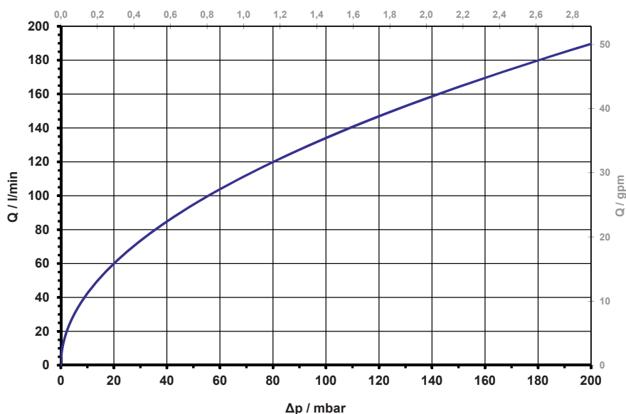
Courbe de débit \Delta p / psi
