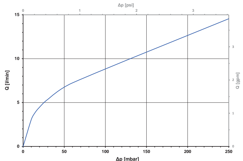
Typische Kennlinie (Vermessung eines Einzelventils unter Laborbedingungen, ohne Regelschraube)
